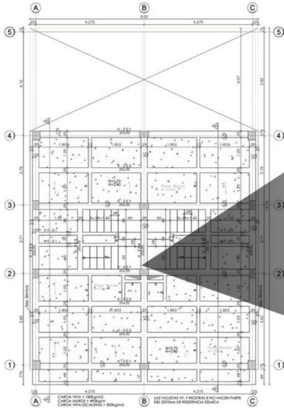
PLANTA PISO 2 Y PISO 3 ESCALA 1:50
