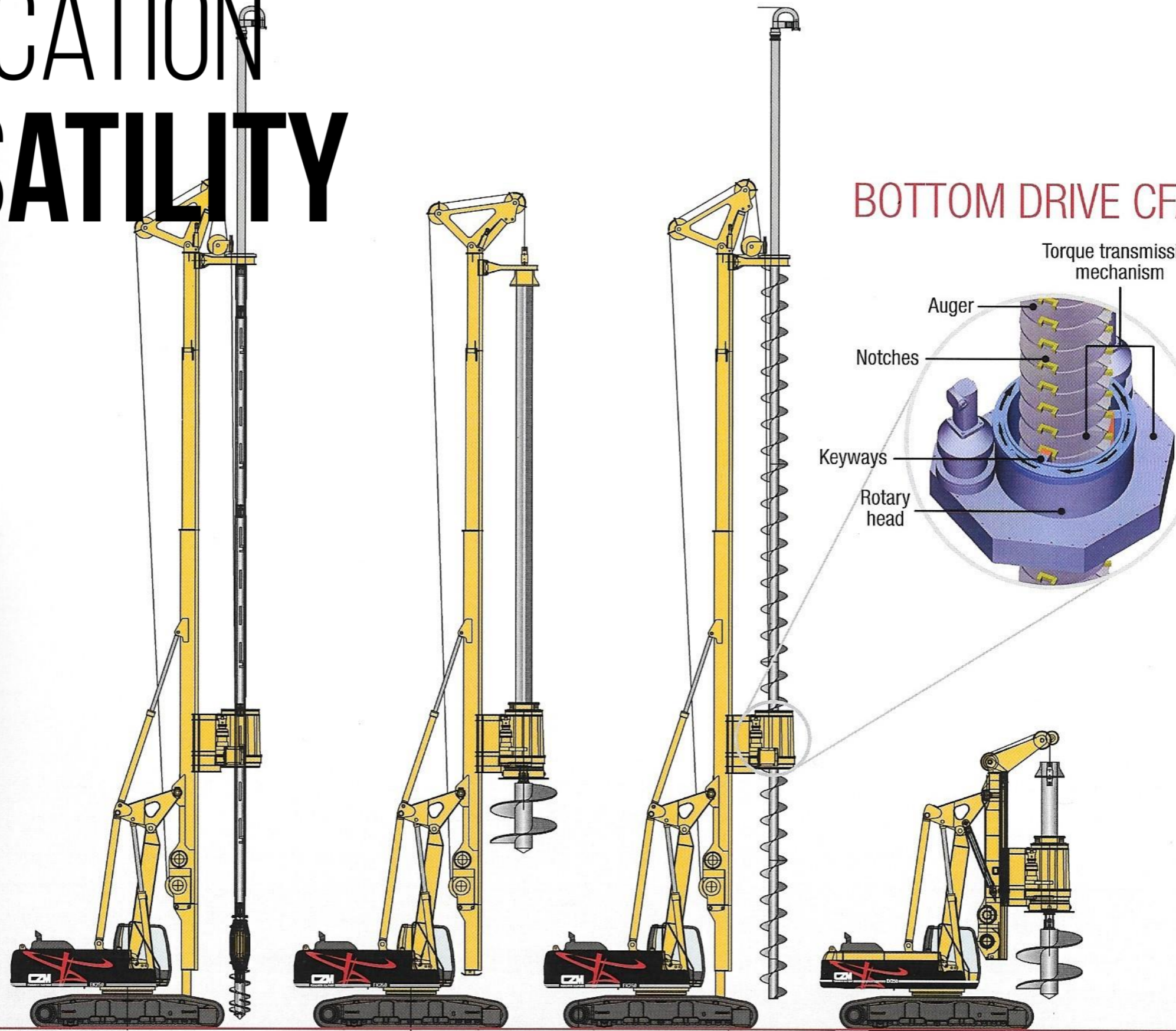
DISPLACEMENT PILE
